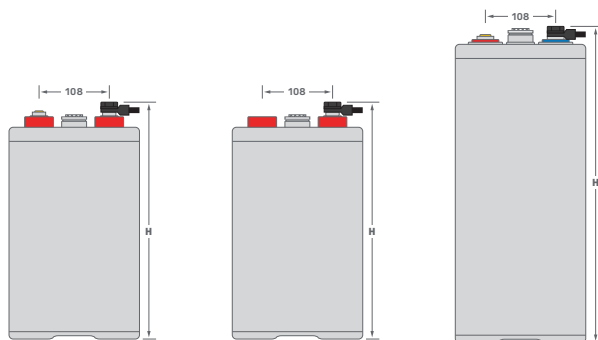
ARG 6V OPzV
